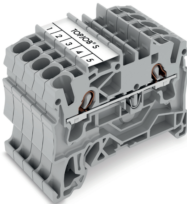
Sorkapocs (2002-1201)
